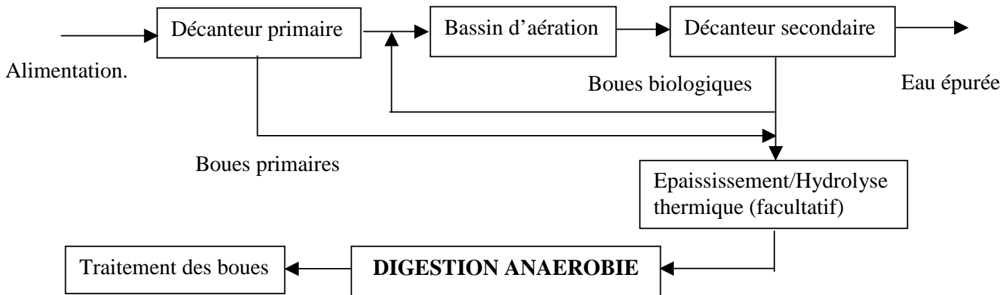
Figure 10 : Circuit du traitement de l'eau d'une station d'épuration urbaine fonctionnant en boues activées.
