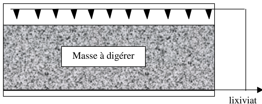
Figure 9 : Exemple de schéma de principe du digesteur à cellules ( fermentation discontinue)
