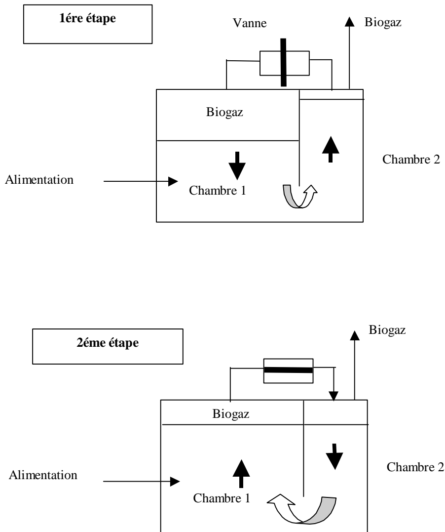
Figure 6 : Schéma de principe d'une agitation générée par le biogaz produit.
