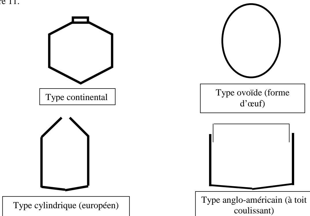
Figure 11 : Différentes formes de digesteurs à boues (Agence de l'eau A.G., Solagro, 2001).
