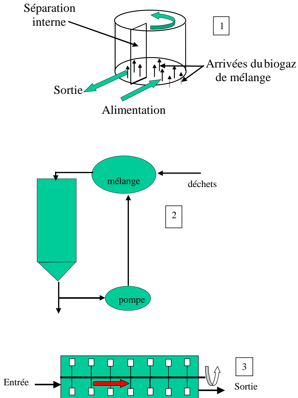
Figure 7 : Schéma de digesteurs en fermentation sèche : 1 Valorga, 2 Dranco, 3 Kompogas.
