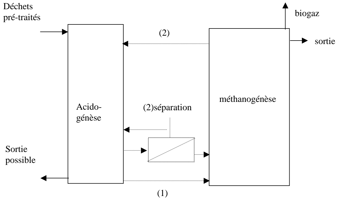
Figure 8 : Stratégies de mise en oeuvre de la digestion anaérobie en deux étapes : (1) couplage direct, (2) séparation des liquides et des solides avec recirculation du lixiviat épuré.
